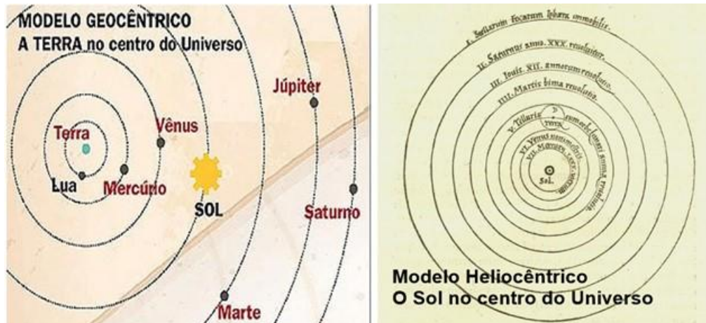
Figura 1: Modelos Heliocêntrico e Geocêntrico. Fonte: Infoescola [11].
