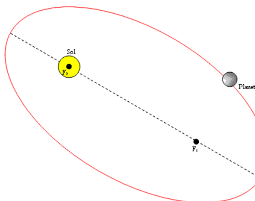
Figura 2: Movimento orbital dos planetas. Fonte: Só Física [12].
